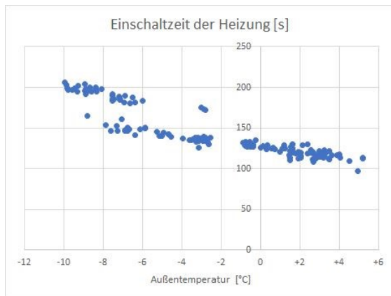
Bild 8: Einschaltzeiten der Heizung bei einer eingestellten Einschalttemperatur von 8^{\circ}\text{C} und einer Ausschalttemperatur von 10^{\circ}\text{C} .
